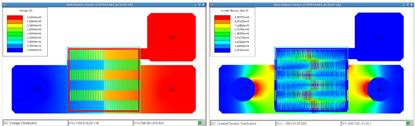
DC Analysis 에 대한 Layout 기반 Contour 분석 제공 (Voltage / Current Density)
