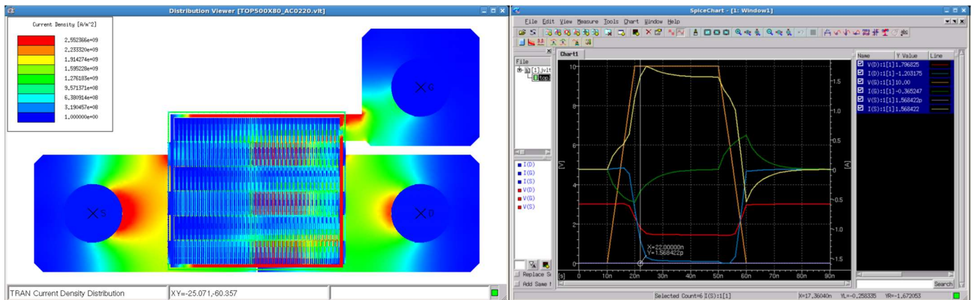
Transient Analysis 에 대한 Layout 기반 Contour 분석 제공
